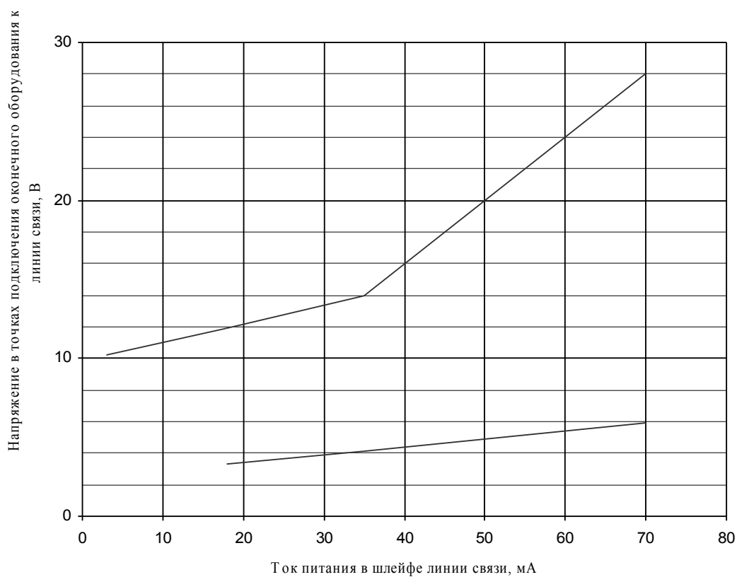
Рисунок П2.1. Зависимость напряжения в точках подключения к линии связи от тока питания в замкнутом шлейфе линии связи
