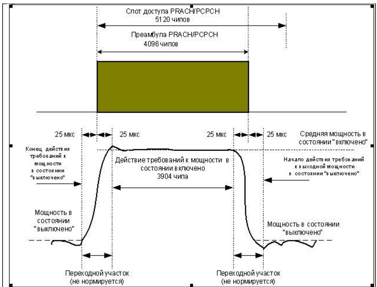
Рисунок 1. Шаблон включения и выключения излучения передатчика во времени для физического канала произвольного доступа
