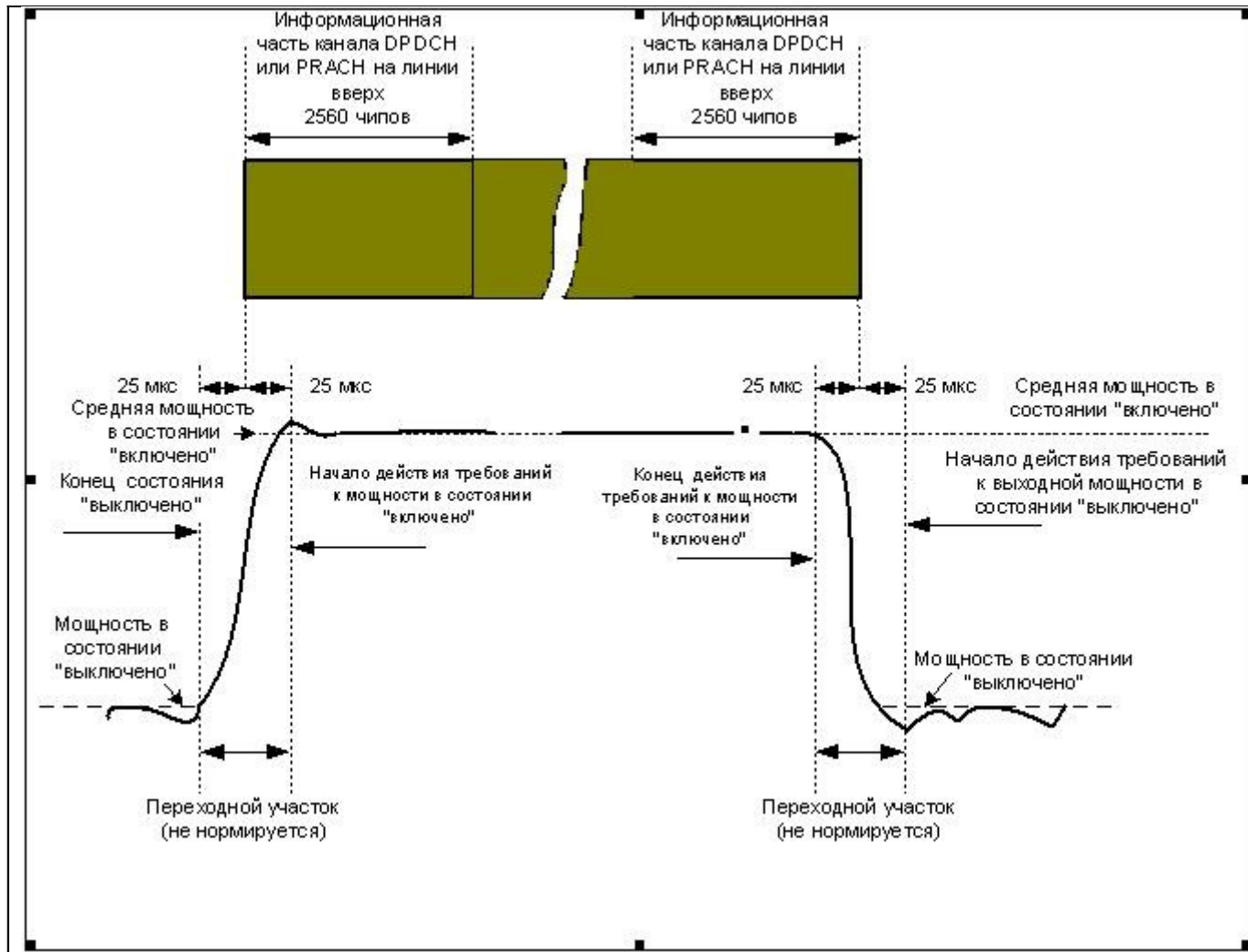
Рисунок 2. Шаблон включения и выключения излучения передатчика во времени для всех остальных каналов
