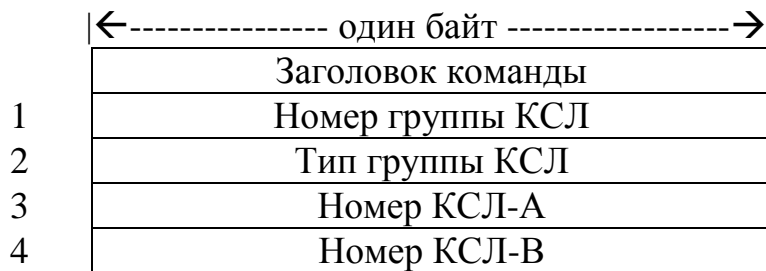
Рисунок 4. Формат команды № 4
