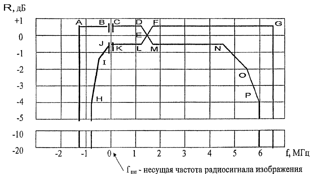
Рисунок 1. Шаблон допустимых значений АЧХ боковых полос в полосе частот от (f - 1,25 \text{ МГц}) до (f + 6,5 \text{ МГц})
