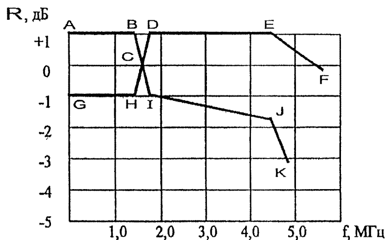
Рисунок 2. Шаблон допустимых значений сквозной АЧХ канала изображения по стандарту В/С (PAL)
